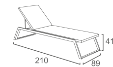
TS-13 TENSE LOUNGER W210 D89 H41 CBM:0.81
