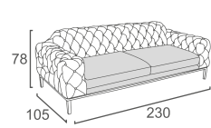
HE-11 HERO 2-S SOFA W230 D105 H78 CBM: 2
